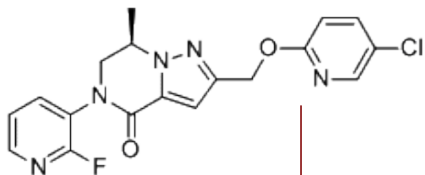
PC-6093601, DMSO-d6
